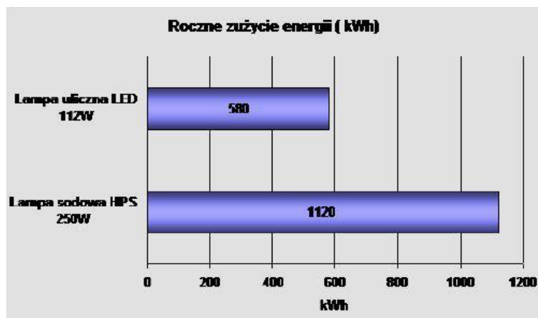
Rys. 4. Zużycie energii elektrycznej lampy sodowej (HPS) i lampy Power LED
