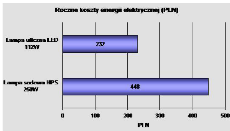
Rys. 5 Zużycie energii elektrycznej lampy sodowej 250 W (HPS) i lampy Power LED 112 W
